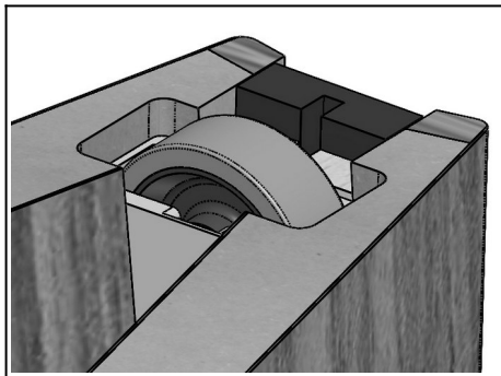
Auszugseite extension side
