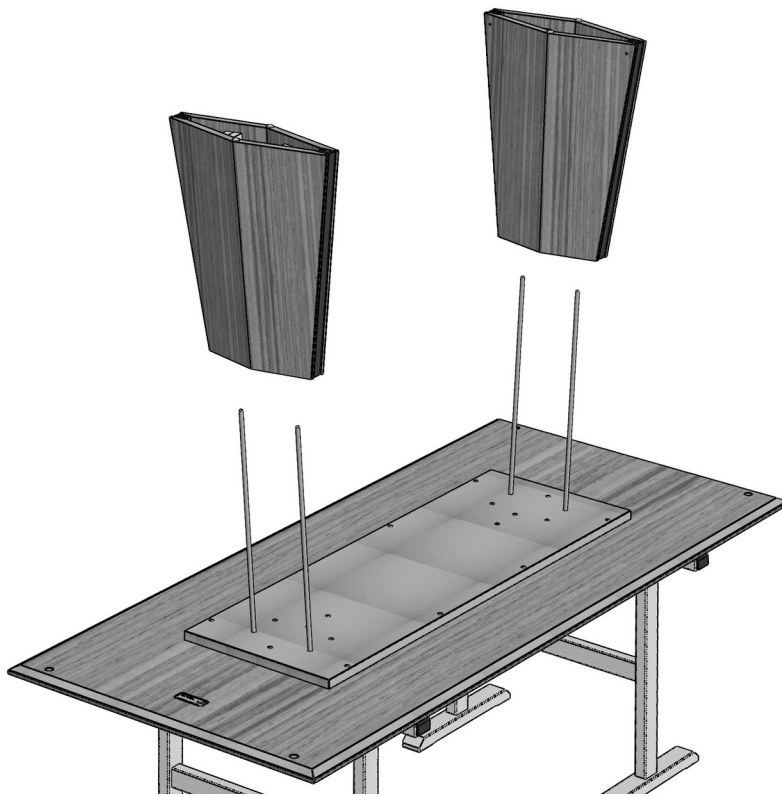
3a. Die beiden Unterbau Wangen aufstecken. 3a. Stick both table feet onto the threaded bolts.
