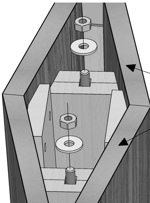
3b. Die beiden Wangen mit Scheiben und Muttern fixieren. 3b. Fix both table feet with washers and nuts.
