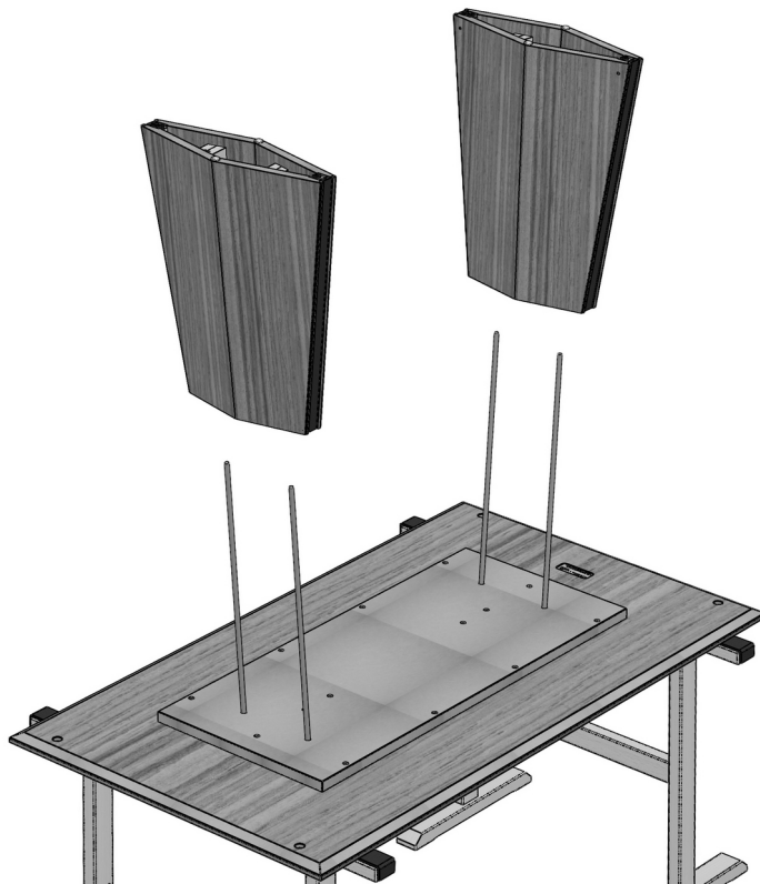
3a. Die beiden Unterbau Wangen aufstecken. 3a. Stick both table feet onto the threaded bolts.
