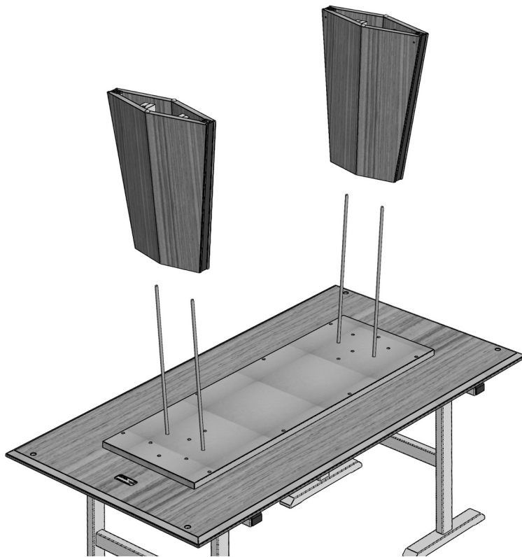
3a. Die beiden Unterbau Wangen aufstecken. 3a. Stick both table feet onto the threaded bolts.
