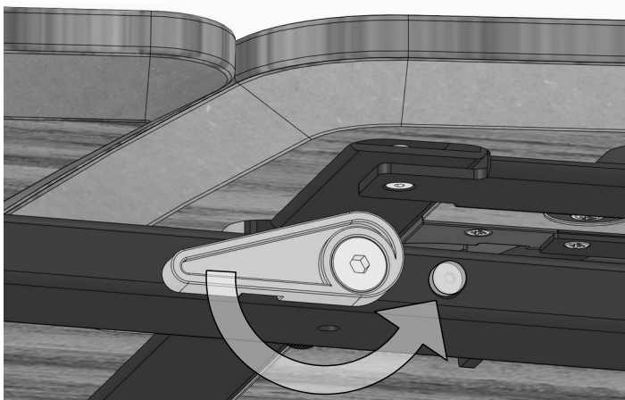
6. Vor dem Ausziehen der Klappeinlage auf der rechten Seite den Bremshebel lösen. 6. Loosen the brake lever on the right side before the extension can be pulled out.
