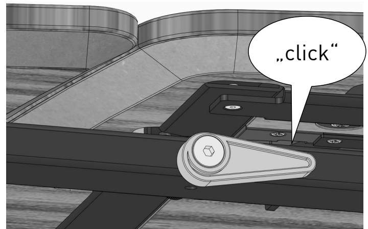
7. Bremse gelöst. Hebel zeigt nach innen und rastet ein. 7. Brake lever released. Lever point inwards and clicks into place.
