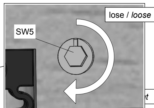
9. Kerbe nach außen: geringe Vorspannung Kerbe nach innen: maximale Vorspannung 9. Notch inwards: low pretension Notch outwards: high pretension
