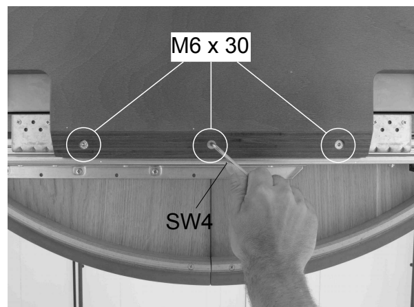
4. ... dass die Bohrungen fluchten. Auf beiden Seiten mit je 3 Inbuschrauben fixieren. 4. ... the holes are lying upon each other. Fix on both sides by using a hex-wrench and each 3 screws.
