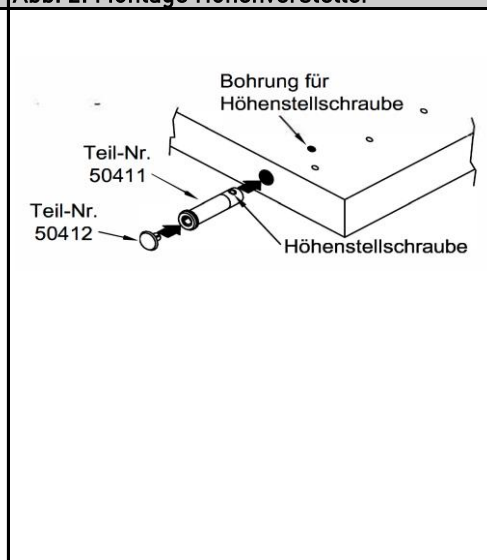
Abb. 2: Montage Höhenversteller
