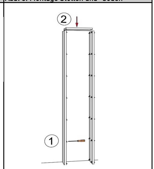
Abb. 3: Montage Stollen und -böden
