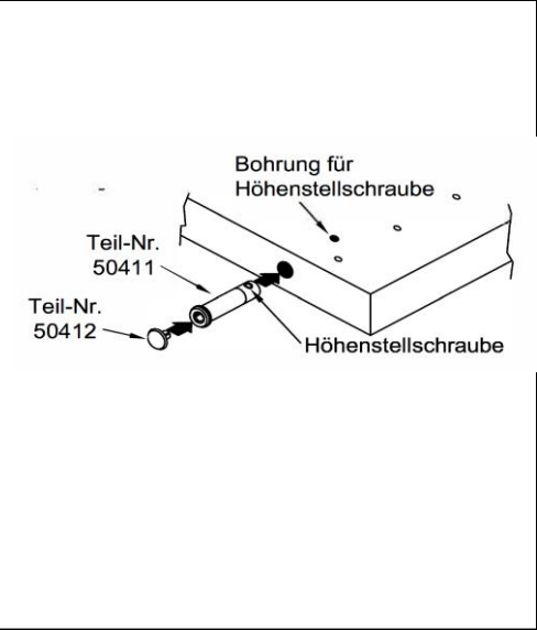
Abb. 2: Montage Höhenversteller
