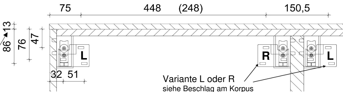
Bohrmaße von Korpus-Außenkante für Aufhängeschienen 60er Element 40er Element
