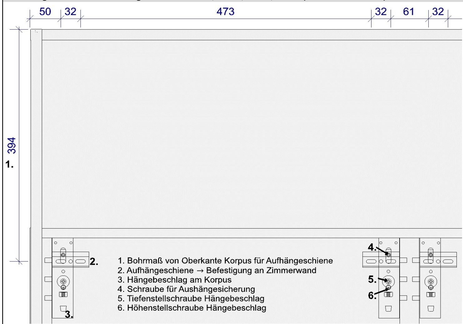
Abbildung 2: Bohrmaße für Hängeelemente W732, W733, W736, W737 (Oben offenes Fach)
