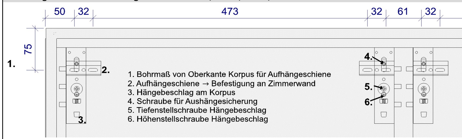
Abbildung 2: Bohrmaße für Hängeelemente W732, W733, W736, W737 (Oben offenes Fach)
