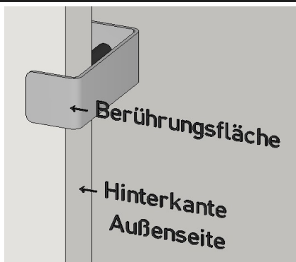
Abbildung 1: Positionierung
