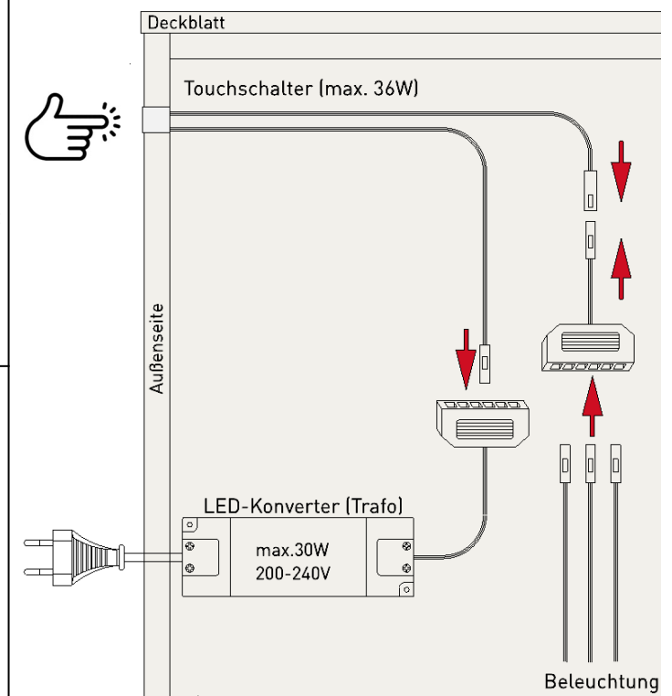
Abbildung 3: Schema Verkabelung
