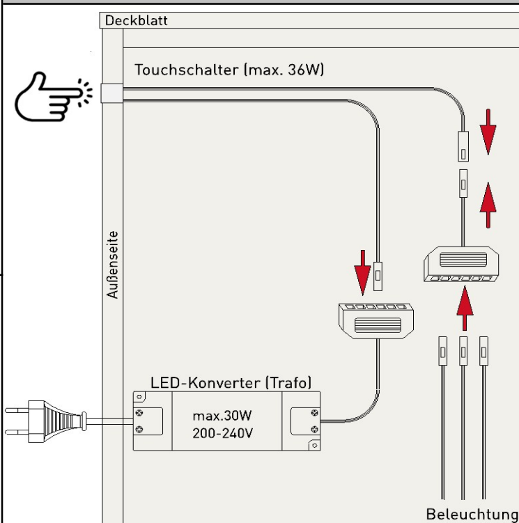
Abbildung 3: Schema Verkabelung
