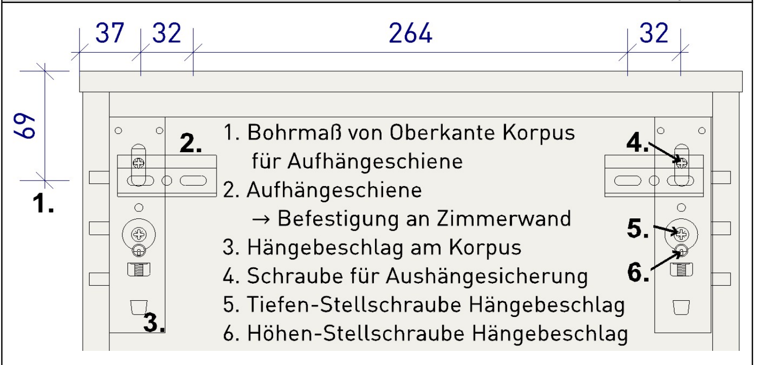
Abbildung 1: Bohrmaße (in mm) von Außenkante Korpus für Aufhängeschienen
