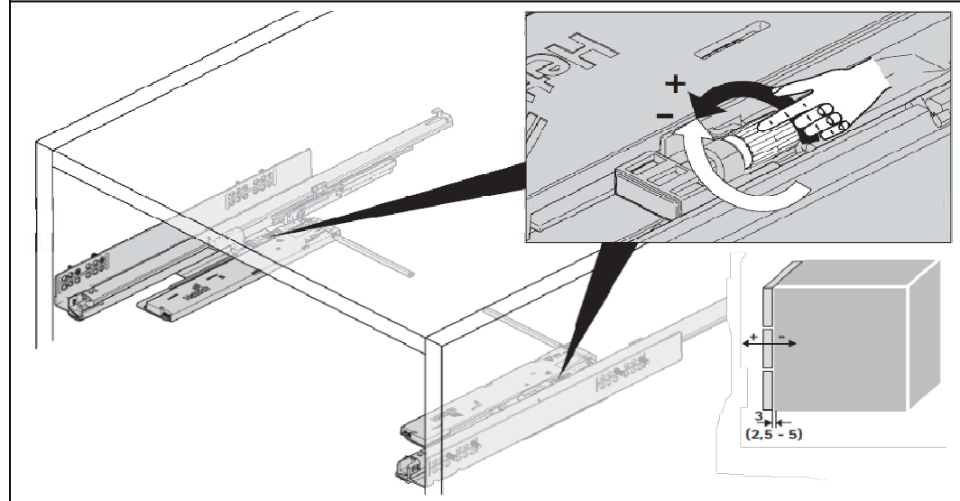
Abbildung 4: Tiefenverstellung
