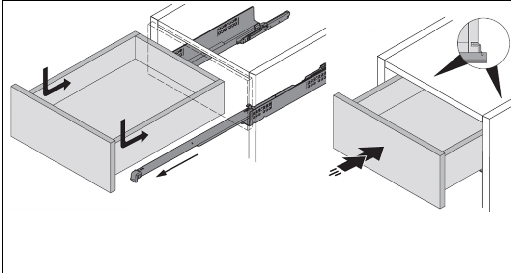
Abbildung 2: Einbau des Schubkasten
