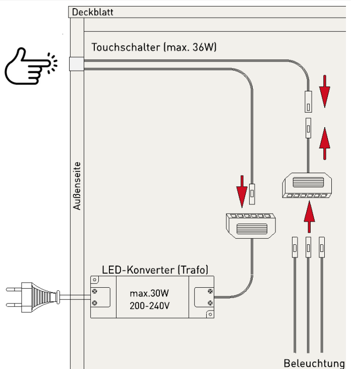
Abbildung 3: Schema Verkabelung
