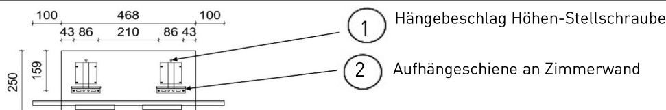
Abbildung 1: Bohrmaße von Außenkante Wandpaneel für Aufhängeschienen
