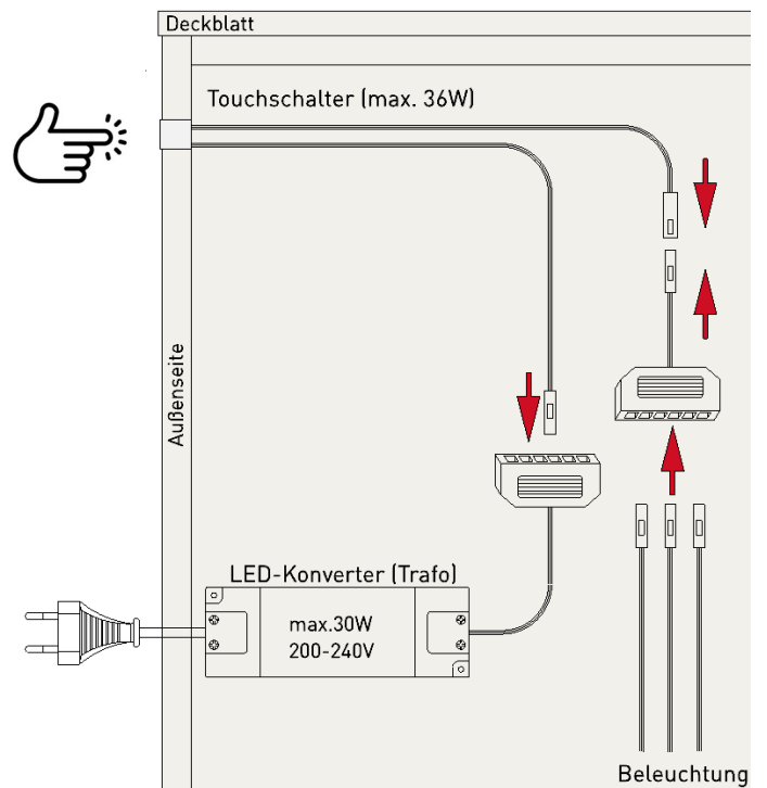
Abbildung 3: Schema Verkabelung
