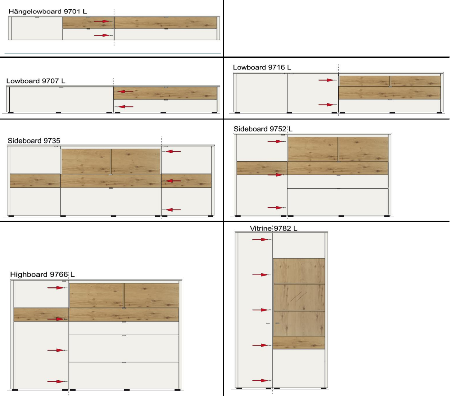
Abbildung 1: Beispiele Korpenverbindung mit Tellerkopfschraube 4x30mm
