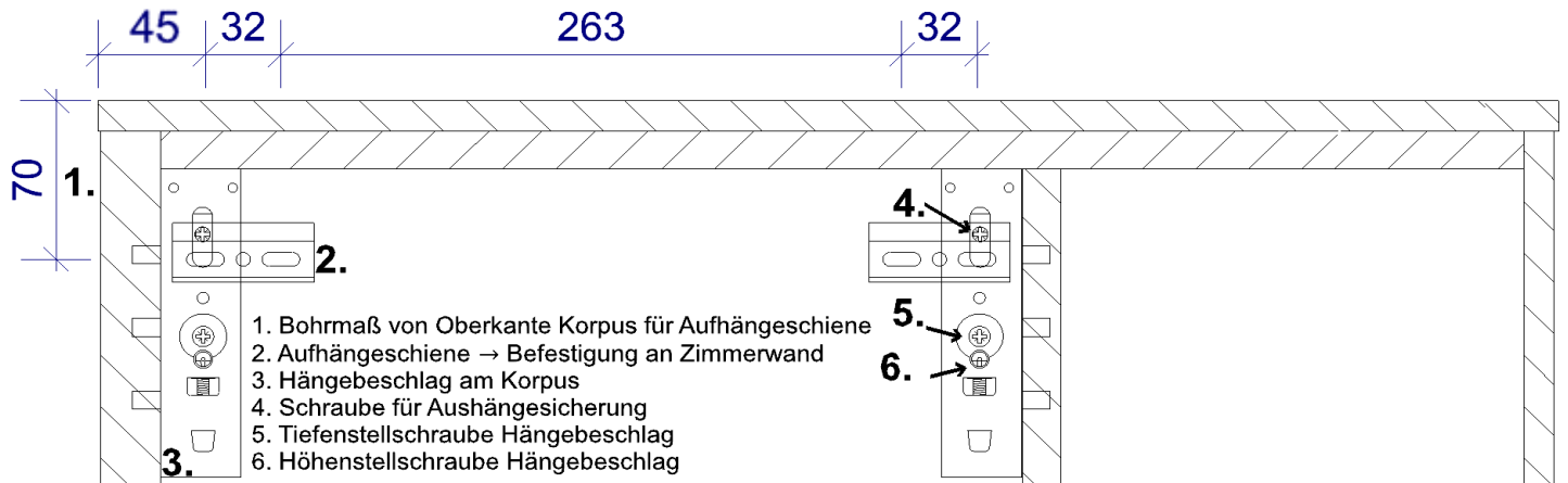
Abbildung 2: Bohrmaße (in mm) von Außenkante Korpus für Aufhängeschienen (Modell 5247)
