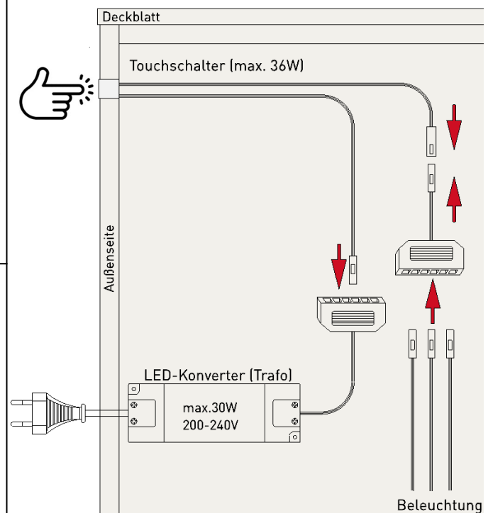
Abbildung 3: Schema Verkabelung
