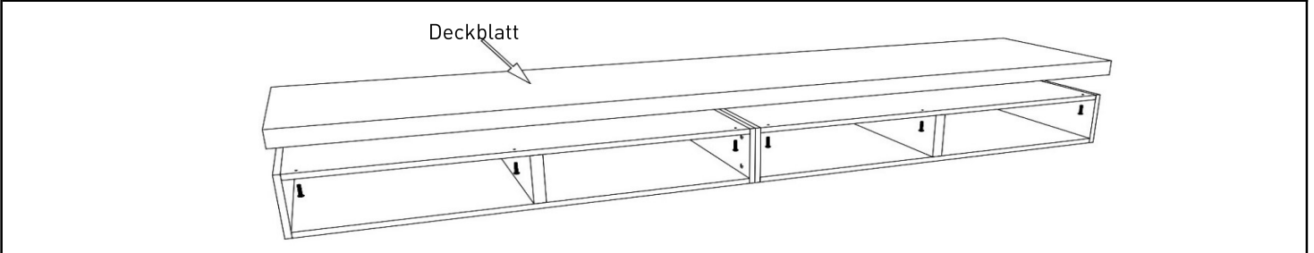
Abbildung 4: Deckblatt festschrauben
