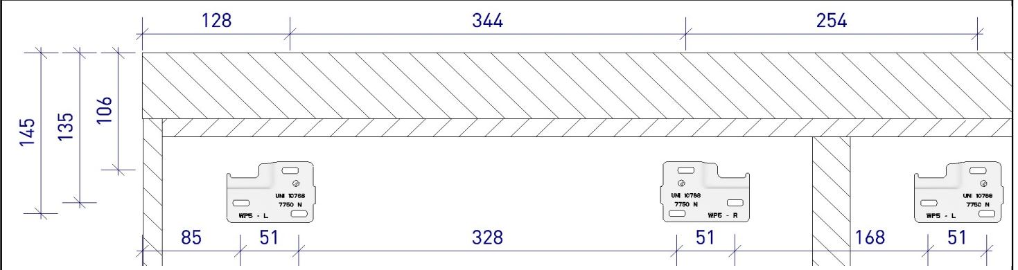
Abbildung 2: Verstellung & Aushängesicherung Hängebeschlag
