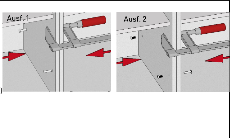
Abbildung 3: Verbindung der Korpusseiten
