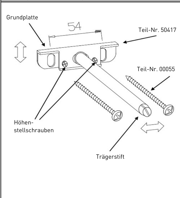
Abbildung 1: Detail Tablarträger
