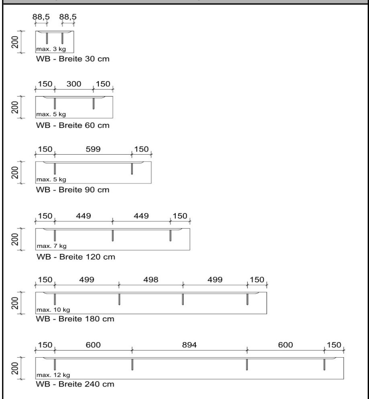
Abbildung 2: Übersicht Wandboardgrößen und Belastbarkeit
