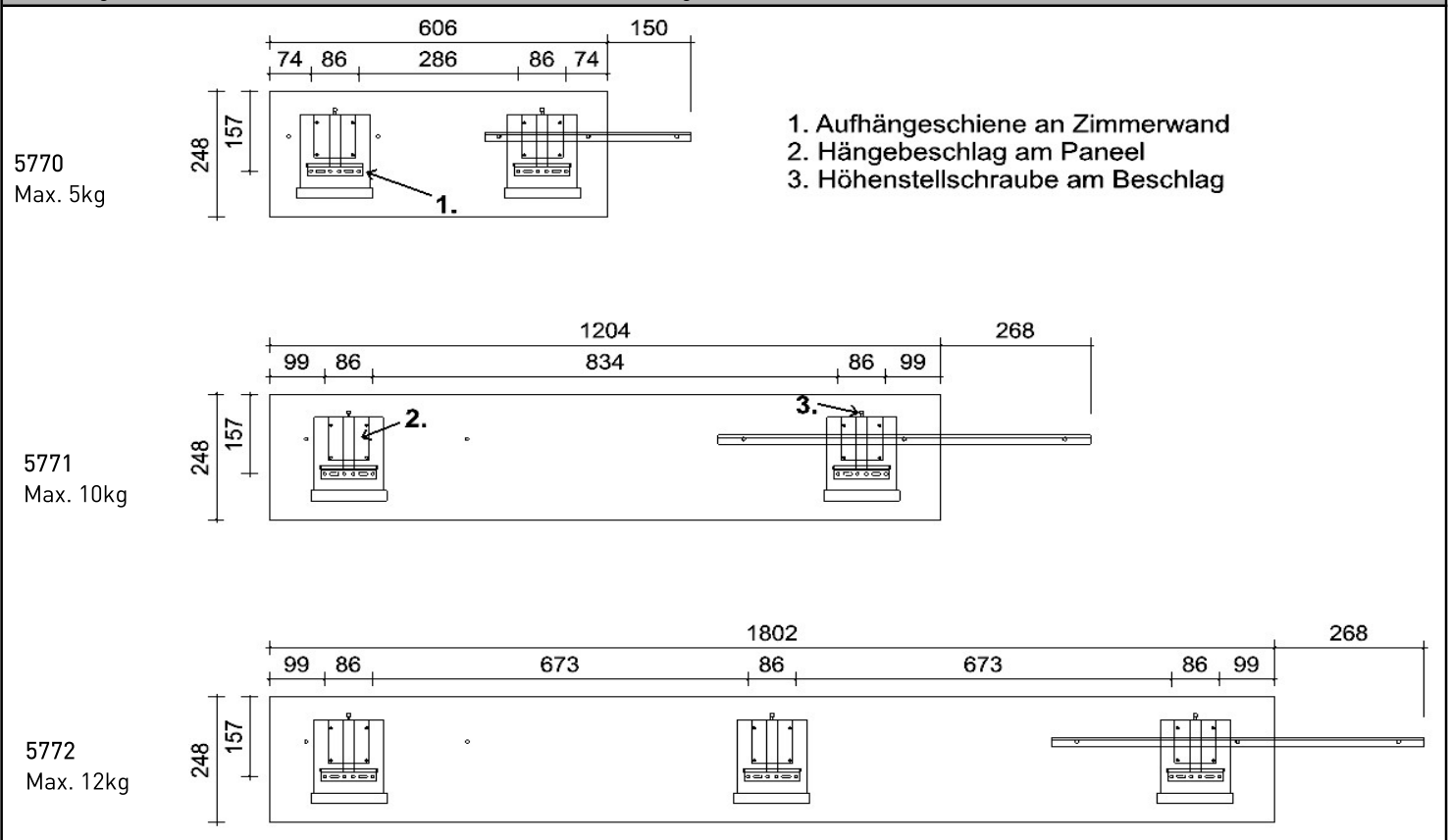
Abbildung 1: Bohrmaße von Wandboard-Außenkanten für Aufhängeschienen
